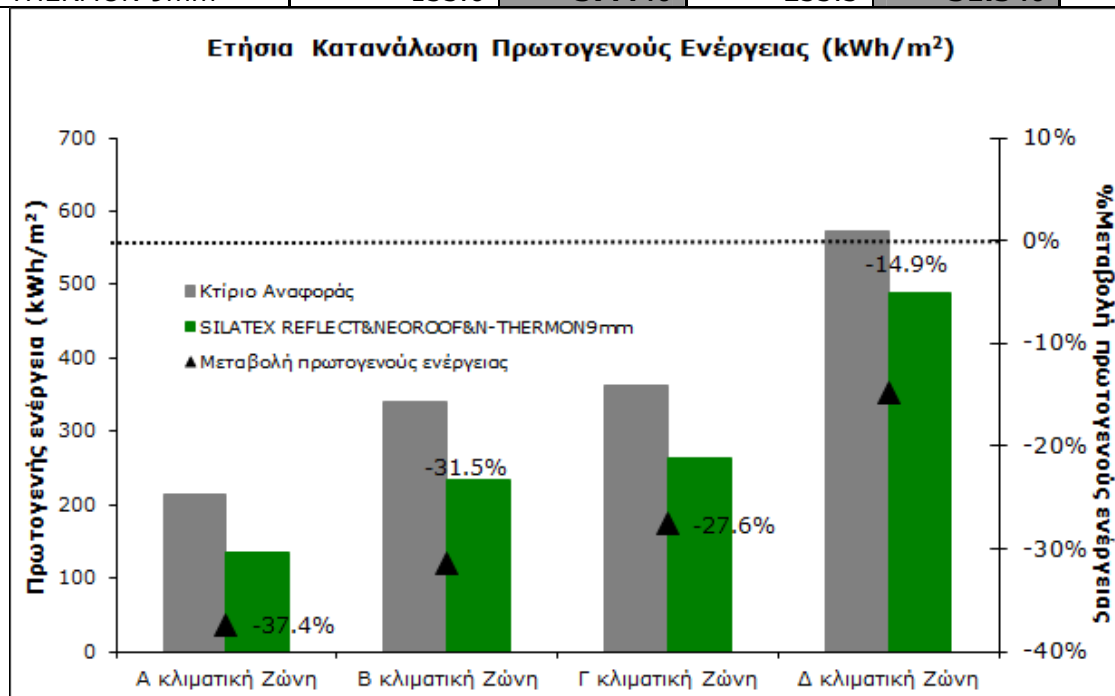
Σχήμα 2 Ετήσια κατανάλωση πρωτογενούς ενέργειας για τη μονοκατοικία πριν (κτίριο αναφοράς) και μετά (SILATEX REFLECT & NEOROOF & N-THERMON 9mm) την εφαρμογή προϊόντων της NEOTEX AEBE.
