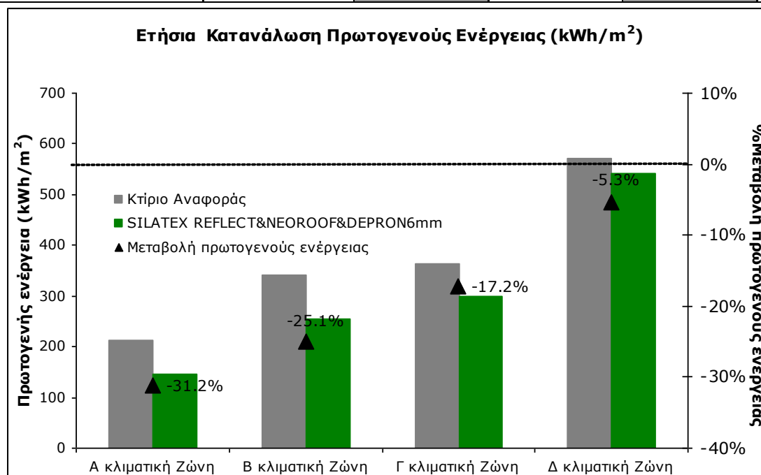
Σχήμα 2 Ετήσια κατανάλωση πρωτογενούς ενέργειας για τη μονοκατοικία πριν (κτίριο αναφοράς) και μετά (SILATEX REFLECT & NEOROOF & DEPRON 6mm) την εφαρμογή προϊόντων της NEOTEX AEBE.
