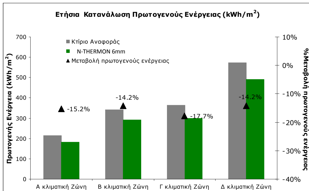
Σχήμα 2 Ετήσια κατανάλωση πρωτογενούς ενέργειας για τη μονοκατοικία πριν (κτίριο αναφοράς) και μετά (N-THERMON 6mm) την εφαρμογή προϊόντων της NEOTEX AEBE .
